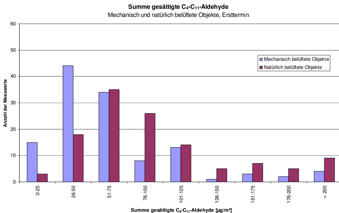
Abb. 4.3.12: Anzahl der Messwerte der Summe der gesättigten azyklischen aliphatischen C 4 -C 11 -Aldehyde in Konzentrationsklassen zu je 25 \mu\text{g}/\text{m}^3 , Wohn- und Schlafräume von Objekten mit Wohnraumlüftungsanlage (n=124) und Objekten mit ausschließlicher Fensterlüftung (n=122), Ersttermin (M1)
