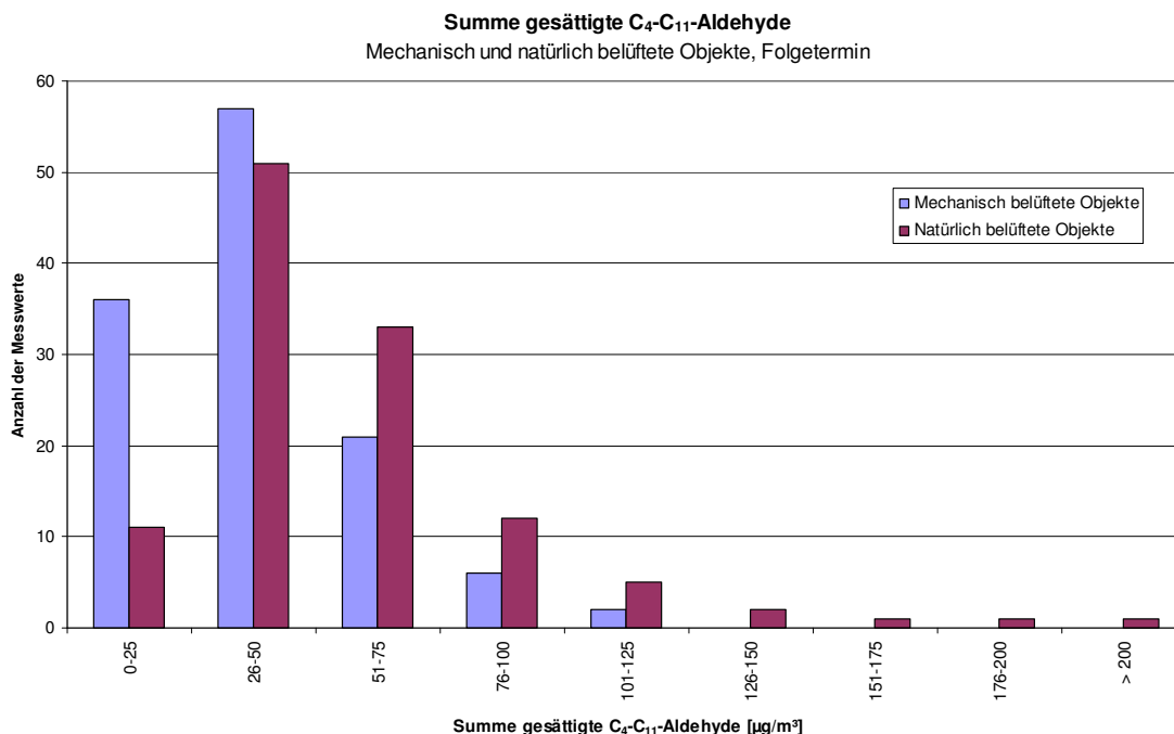
Abb. 4.3.13: Anzahl Messwerte der Summe der gesättigten azyklischen aliphatischen C 4 -C 11 -Aldehyde in Konzentrationsklassen zu je 25 \mu\text{g}/\text{m}^3 , Wohn- und Schlafräume von Objekten mit Wohnraumlüftungsanlage (n=122) und Objekten mit ausschließlicher Fensterlüftung (n=117), Folgetermin (M2)
