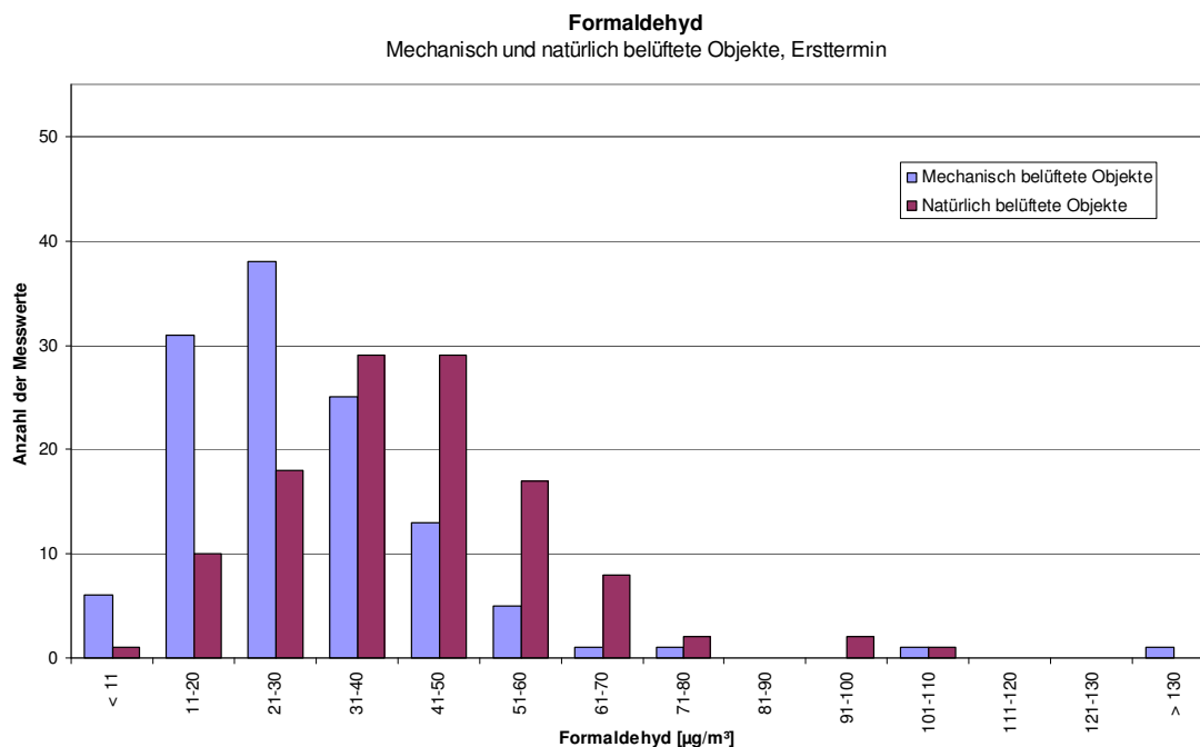
Abb. 4.3.7: Anzahl der Formaldehyd-Messwerte in Konzentrationsklassen zu je 10 \mu\text{g}/\text{m}^3 , Wohn- und Schlafräume in Objekten mit Wohnraumlüftungsanlage (n=122) und in Objekten mit ausschließlicher Fensterlüftung (n=117), Ersttermin (M1)
