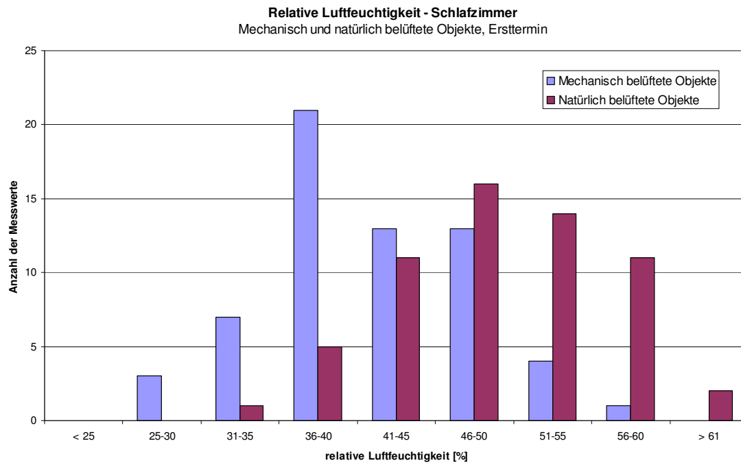
Abb. 4.3.19: Anzahl der der relativen Luftfeuchtigkeits-Werte in Konzentrationsklassen zu je 5 % in den Schlafräumen von Objekten mit Wohnraumlüftungsanlagen (n=62) und mit ausschließlicher Fensterlüftung (n=60), Ersttermin (M1)
