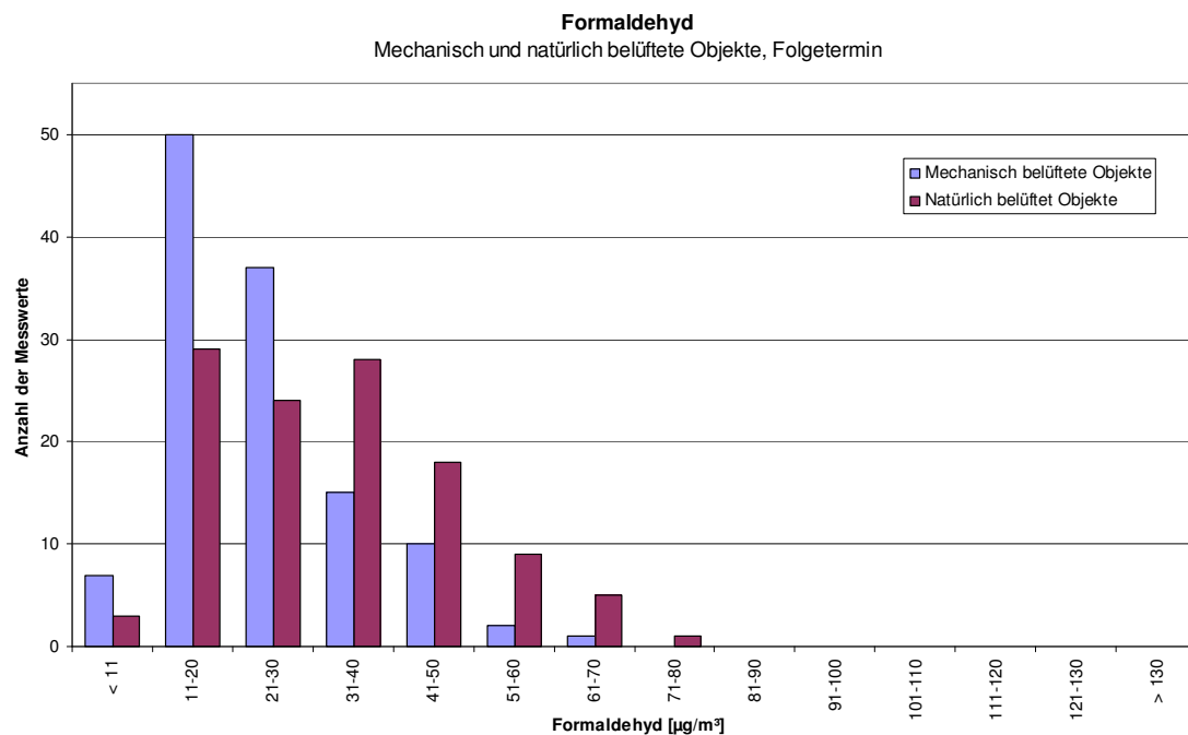
Abb. 4.3.8: Anzahl der Formaldehyd-Messwerte in Konzentrationsklassen zu je 10 µg/m³, Wohn- und Schlafräume in Objekten mit Wohnraumlüftungsanlage (n=122) und in Objekten mit ausschließlicher Fensterlüftung (n=117), Folgetermin (M2)
