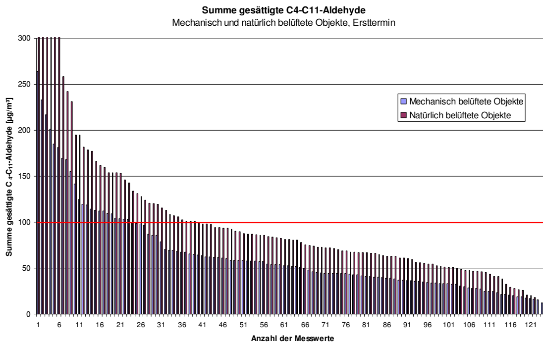
Abb. 3.5.26: Summe gesättigter azyklischer aliphatischer C 4 -C 11 -Aldehyde in Wohn- und Schlafräumen von Objekten mit Wohnraumlüftungsanlage sowie von Objekten mit ausschließlicher Fensterlüftung, Ersttermin (M1)
