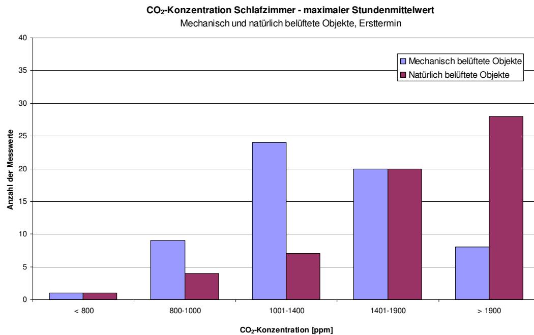
Abb. 4.3.16: Anzahl der CO 2 -Messwerte (maximaler gleitender Stundenmittelwert) in Konzentrationsklassen laut Akademie der Wissenschaften/BMLFUW (2011) bzw. ÖNORM EN 13779, Schlafräume von Objekten mit Wohnraumlüftungsanlagen (n=62) und mit ausschließlicher Fensterlüftung (n=60), Ersttermin (M1)
