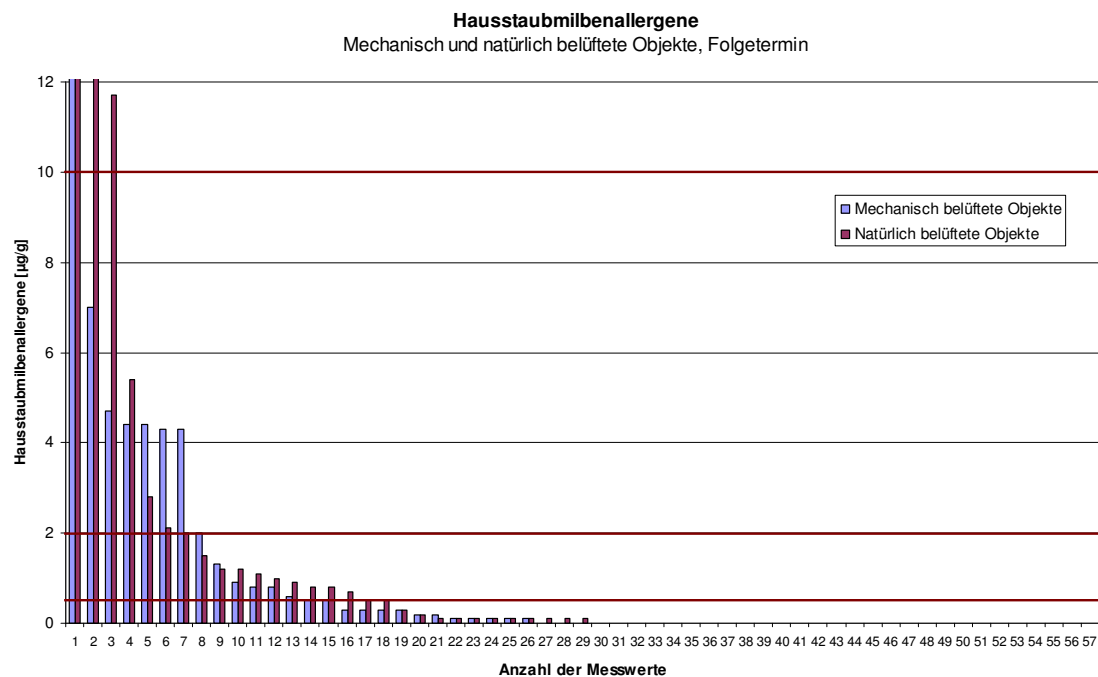
Abb. 3.5.40: Summe der Konzentration an Der p1 und Der p2 in Wohn- und Schlafräumen der Objekte mit Wohnraumlüftungsanlage sowie der Objekte mit ausschließlicher Fensterlüftung, Folgetermin (M2)
