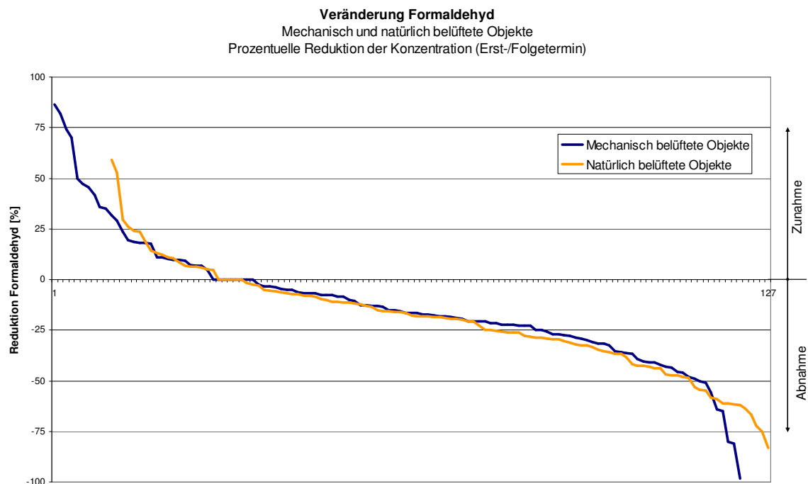
Abb. 3.5.23: Prozentuelle Reduktion der Formaldehyd-Werte in Wohn- und Schlafräumen von Objekten mit Wohnraumlüftungsanlage sowie von Objekten mit ausschließlicher Fensterlüftung zwischen beiden Messterminen (M1, M2)
