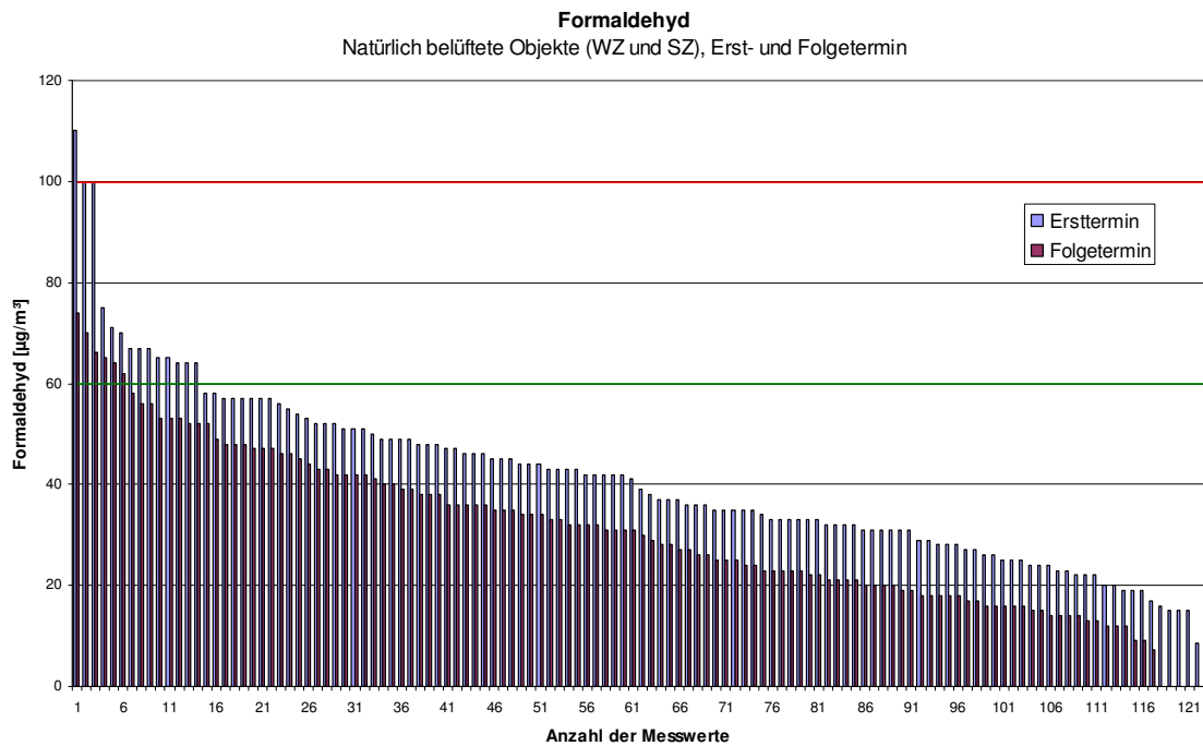
Abb. 3.5.20: Formaldehyd-Konzentrationen in Wohn- und Schlafräumen von Objekten mit ausschließlicher Fensterlüftung, Erst- und Folgetermin (M1, M2)
