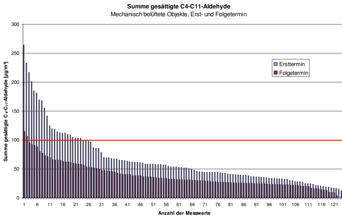
Abb. 3.5.24: Summe gesättigter azyklischer aliphatischer C 4 -C 11 -Aldehyde in Wohn- und Schlafräumen von Objekten mit Wohnraumlüftungsanlage, Erst- und Folgetermin (M1, M2)
