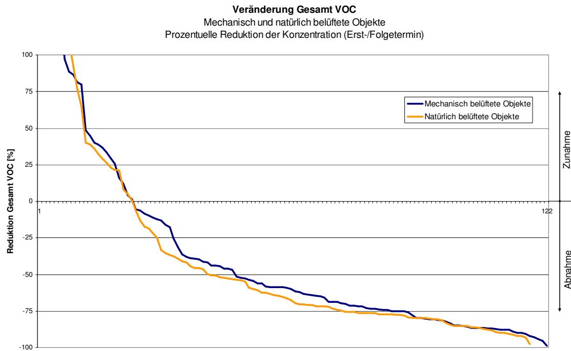
Abb. 3.5.13: Prozentuelle Veränderung der Gesamt VOC-Werte in Wohn- und Schlafräumen von Objekten mit Wohnraumlüftungsanlage sowie von Objekten mit ausschließlicher Fensterlüftung zwischen beiden Messterminen (M1, M2)
