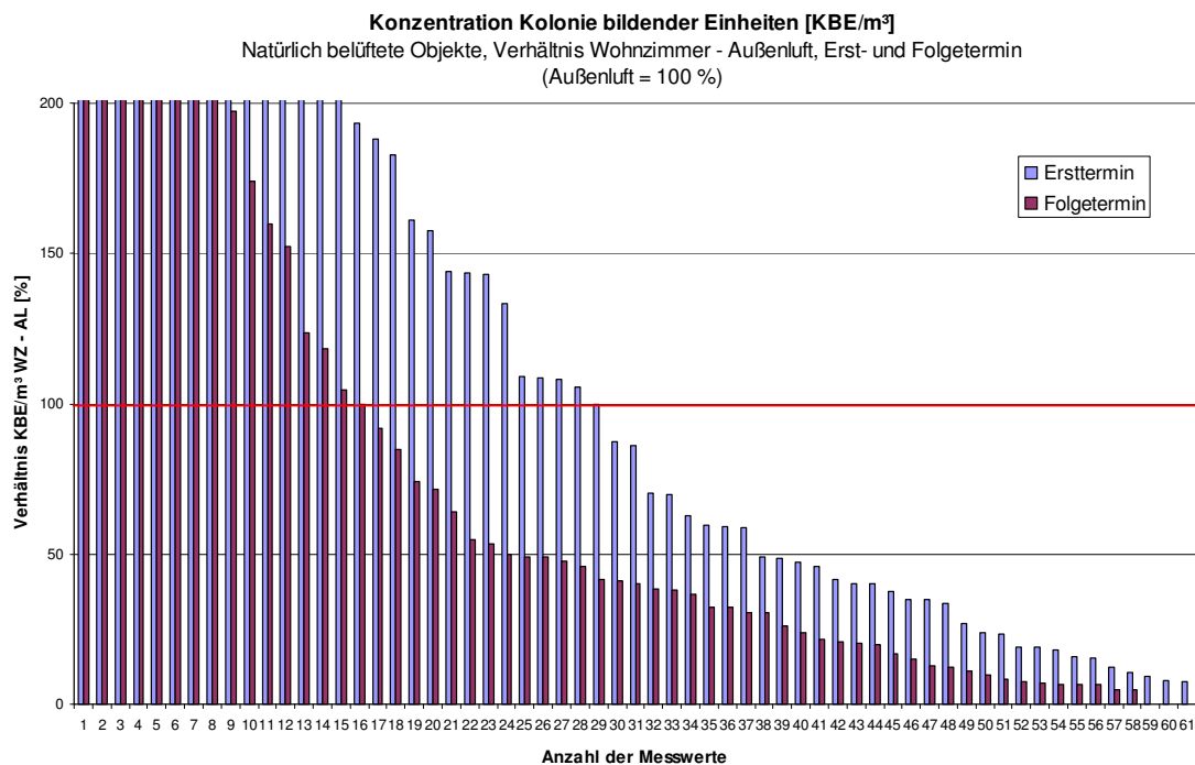
Abb. 3.5.31: Verhältnis der Konzentration an KBE/m 3 in den Wohnräumen der Objekte mit ausschließlicher Fensterlüftung und der Außenluft, Erst- und Folgetermin (M1, M2)
