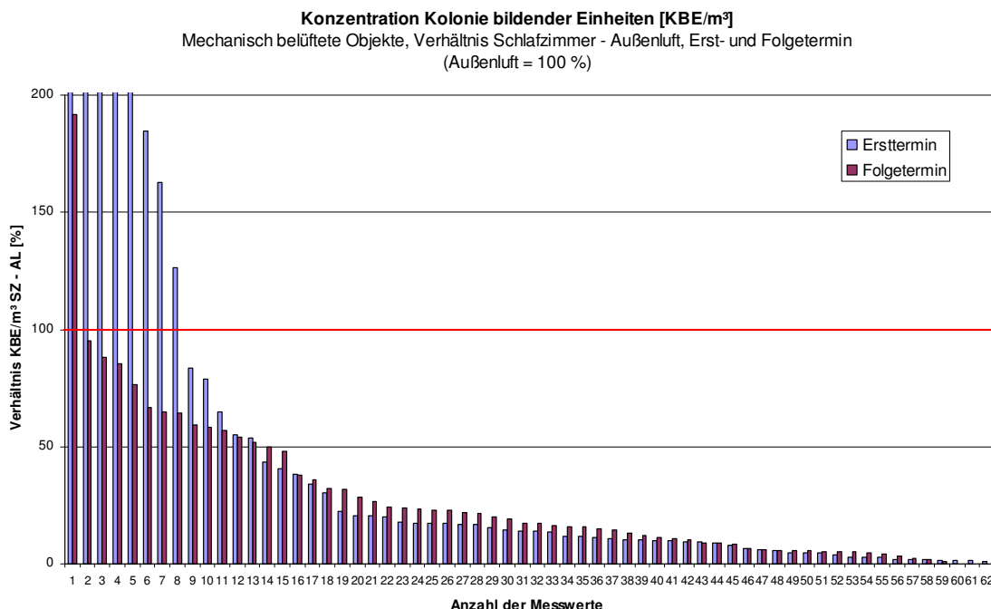
Abb. 3.5.28: Verhältnis der Konzentration an KBE/m 3 in den Schlafräumen der Objekte mit Wohnraumlüftungsanlage und der Außenluft, Erst- und Folgetermin (M1, M2)
