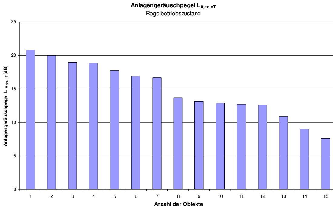
Abb. 3.5.58: Differenz des äquivalenten Anlagengeräuschpegels zwischen ausgeschalteter Anlage und Regelbetriebszustand (Stufe 2) in den Schlafräumen der Objekte mit Wohnraumlüftungsanlage, Ersttermin (M1). Es ist ersichtlich, dass für den Regelbetriebszustand alle Lüftungsanlagen sowohl die baugesetzlichen Anforderung als auch die Qualitätsstandards von komfortlüftung.at eingehalten werden
