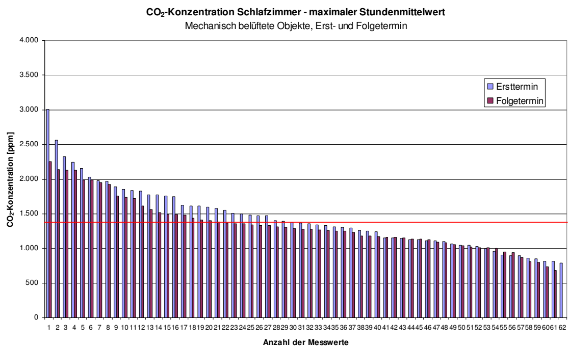
Abb. 3.5.48: CO 2 -Konzentration (max. gleitender Stundenmittelwert) im Schlafräum der Objekte mit Wohnraumlüftungsanlage, Erst- und Folgetermin (M1, M2)
