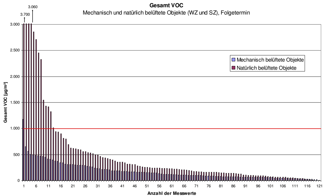
Abb. 3.5.4: Gesamt VOC-Werte in Wohn- und Schlafräumen von Objekten mit Wohnraumlüftungsanlage sowie von Objekten mit ausschließlicher Fensterlüftung, Folgetermin (M2)
