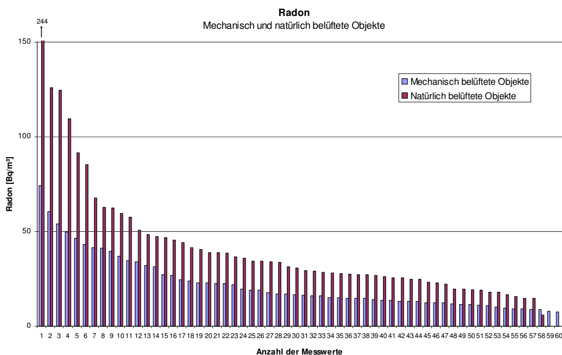
Abb. 3.5.56: Radon-Konzentration in Objekten mit Wohnraumlüftungsanlage sowie in Objekten mit ausschließlicher Fensterlüftung, arithmetischer Mittelwert der Konzentrationen im jeweiligen Objekt
