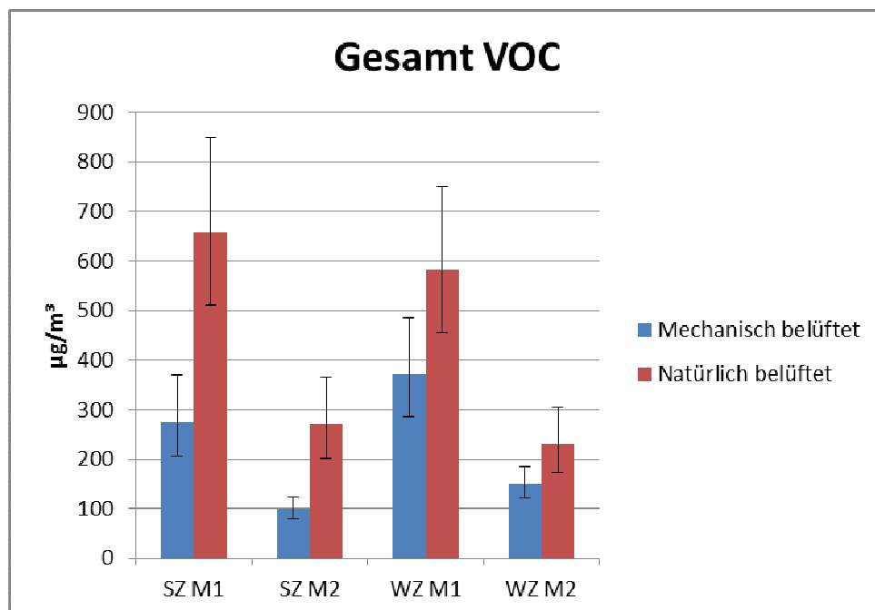
Abb. 4.3.5: Gesamt VOC-Werte in Wohn- (WZ) und Schlafräumen (SZ) in Objekten mit Wohnraumlüftungsanlage sowie in Objekten mit ausschließlicher Fensterlüftung, Erst- und Folgetermin (M1, M2), geometrische Mittelwerte und 95 % Konfidenzintervalle
