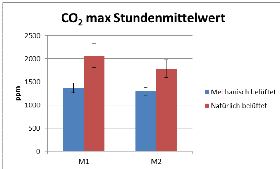
Abb. 4.3.18: CO 2 -Konzentration (maximaler gleitender Stundenmittelwert) im Schlafraum von Objekten mit und ohne Wohnraumlüftungsanlagen, Erst- und Folgetermin (M1, M2), geometrische Mittelwerte und 95 % Konfidenzintervalle
