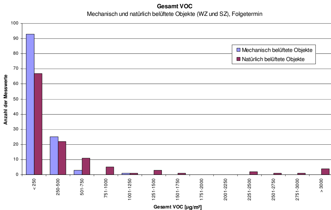
Abb. 4.3.4: Anzahl der Gesamt VOC- Messwerte in Konzentrationsklassen zu je 250 µg/m 3 , Wohn- und Schlafräume von Objekten mit Wohnraumlüftungsanlage (n=122) und Objekten mit ausschließlicher Fensterlüftung (n=118) Objekte, Folgetermin (M2)
