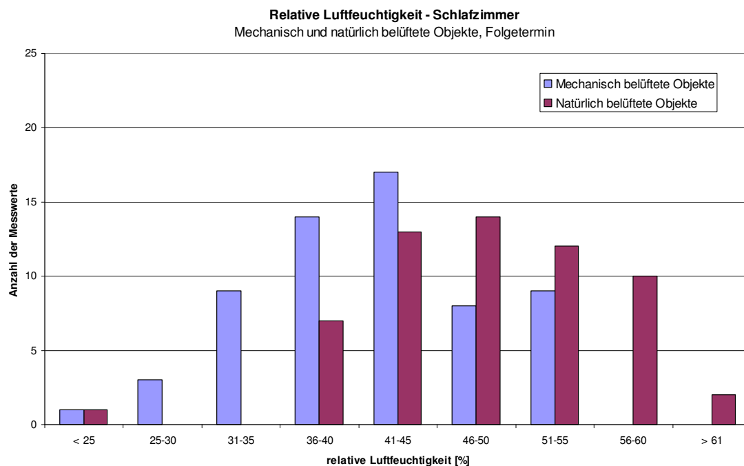
Abb. 4.3.20: Anzahl der der relativen Luftfeuchtigkeits-Werte in Konzentrationsklassen zu je 5 % in den Schlafräumen mit Wohnraumlüftungsanlagen (n=61) und mit ausschließlicher Fensterlüftung (n=59), Folgetermin (M2)
