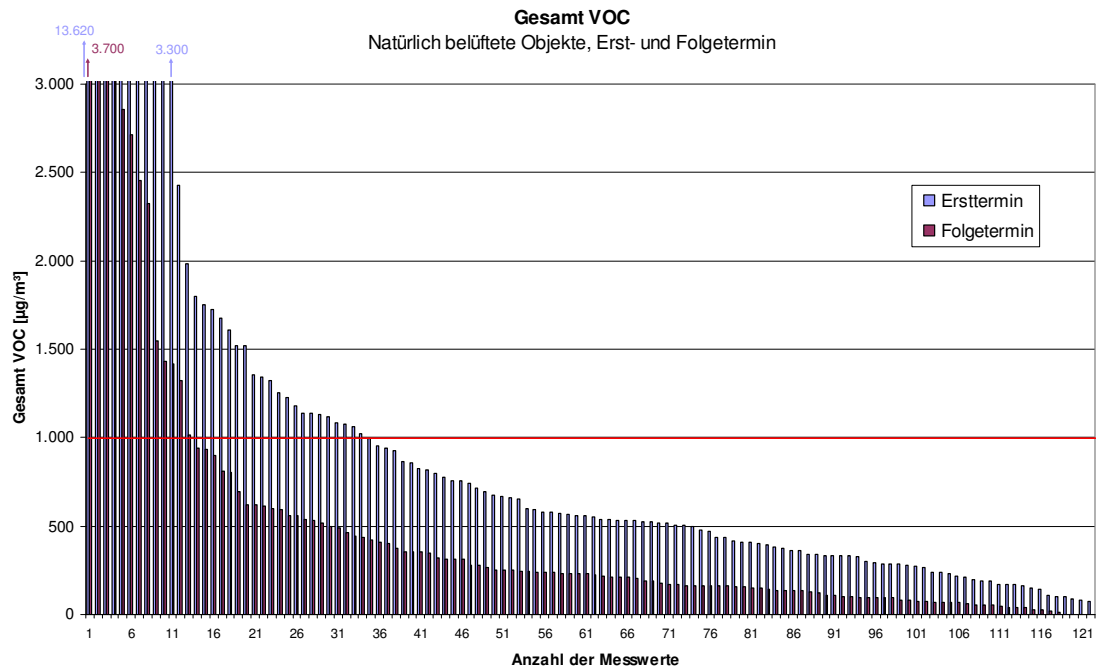
Abb. 3.5.2: Gesamt VOC-Werte in Wohn- und Schlafräumen von Objekten mit ausschließlicher Fensterlüftung, Erst- und Folgetermin (M1, M2)
