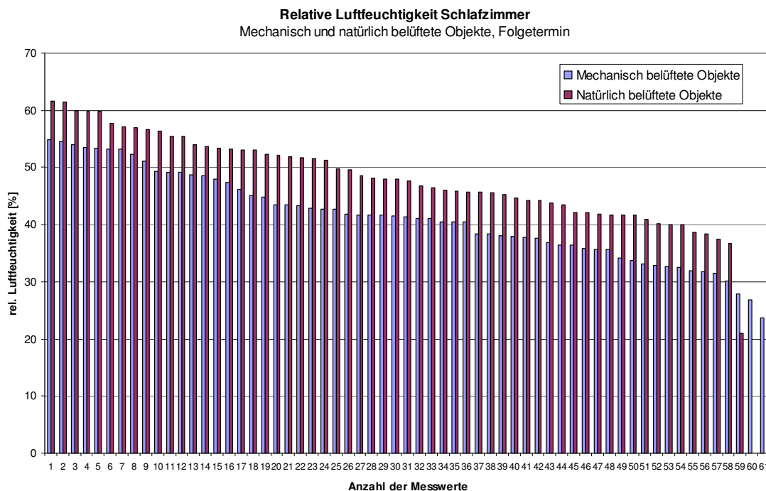
Abb. 3.5.63: Relative Luftfeuchtigkeit im Schlafraum der Objekte mit Wohnraumlüftungsanlage sowie der Objekte mit ausschließlicher Fensterlüftung, arithmetischer Mittelwert über den Zeitraum einer Woche, Folgetermin (M2)
