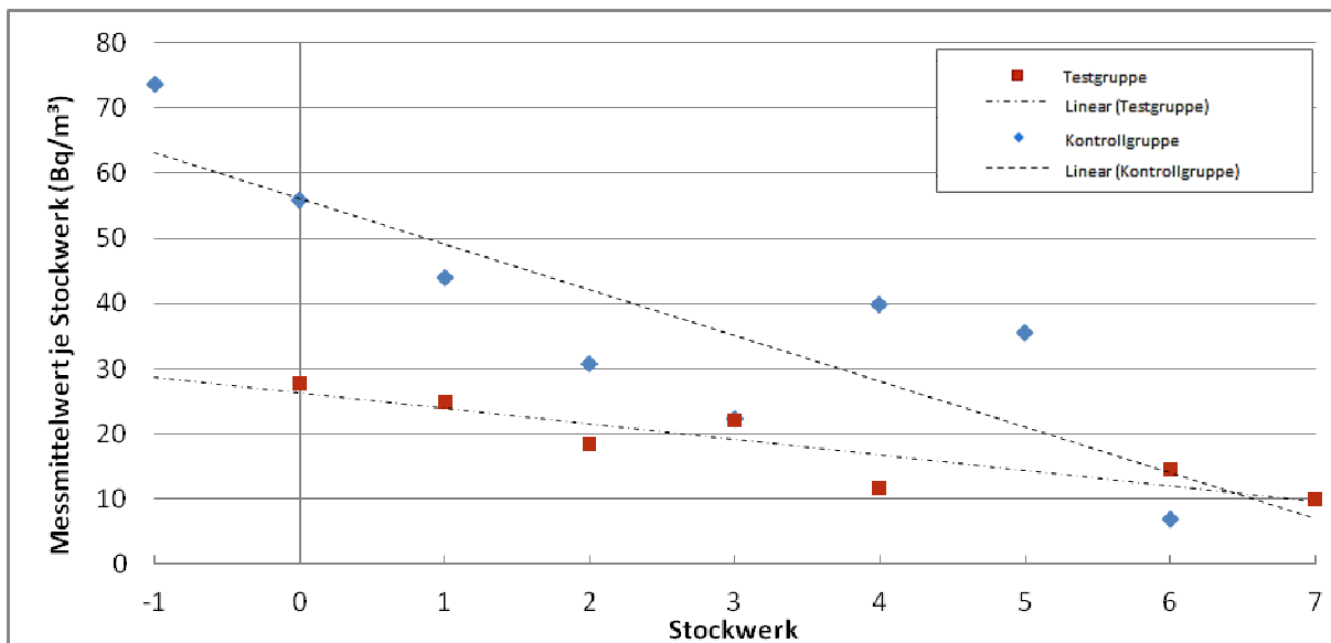
Abb. 8.7: Abnahme der Radonkonzentration mit steigendem Stockwerk, angegeben werden die arithmetischen Mittelwerte der Gebäudemittelwerte
