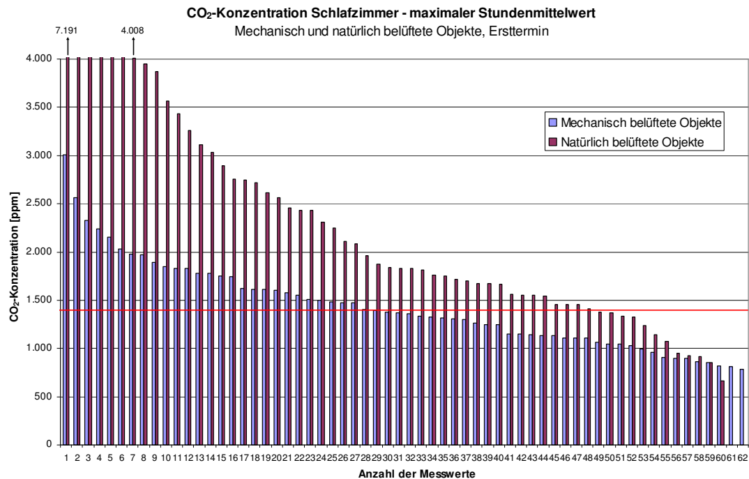
Abb. 3.5.50: CO 2 -Konzentration (max. gleitender Stundenmittelwert) im Schlafrum der Objekte mit Wohnraumlüftungsanlage sowie der Objekte mit ausschließlicher Fensterlüftung, Ersttermin (M1)
