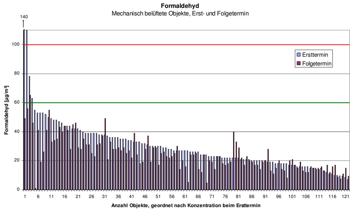
Abb. 4.3.10: Formaldehyd-Konzentrationen in Wohn- und Schlafräumen der Objekte mit Wohnraumlüftungsanlage, Erst- und jeweils zugeordneter Folgetermin (M1, M2), Veränderung der Konzentrationen, geordnet nach Konzentrationen bei Ersttermin
