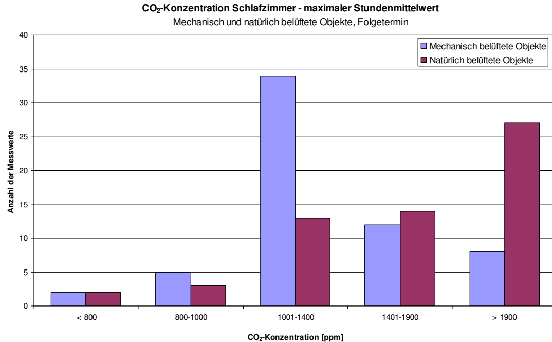
Abb. 4.3.17: Anzahl der CO 2 -Messwerte (maximaler gleitender Stundenmittelwert) in Konzentrationsklassen laut Akademie der Wissenschaften/BMLFUW (2011) bzw. ÖNORM EN 13779, Schlafräume von Objekten mit Wohnraumlüftungsanlagen (n=61) und mit ausschließlicher Fensterlüftung (n=59), Folgetermin (M2)
