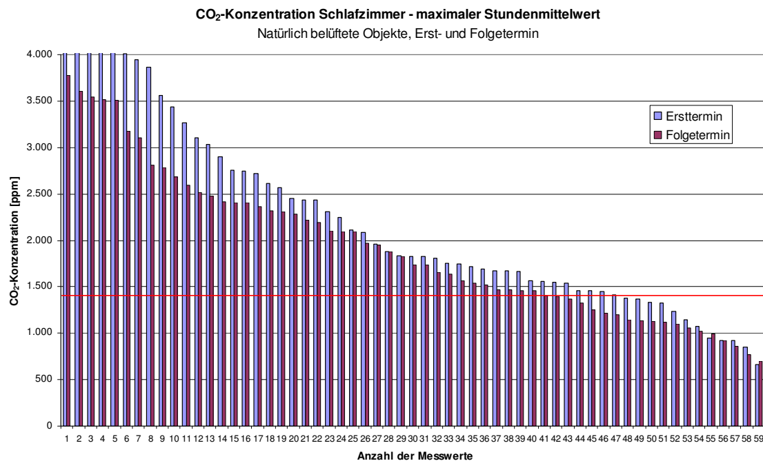
Abb. 3.5.49: CO 2 -Konzentration (max. gleitender Stundenmittelwert) im Schlafrum der Objekte mit ausschließlicher Fensterlüftung, Erst- und Folgetermin (M1, M2)
