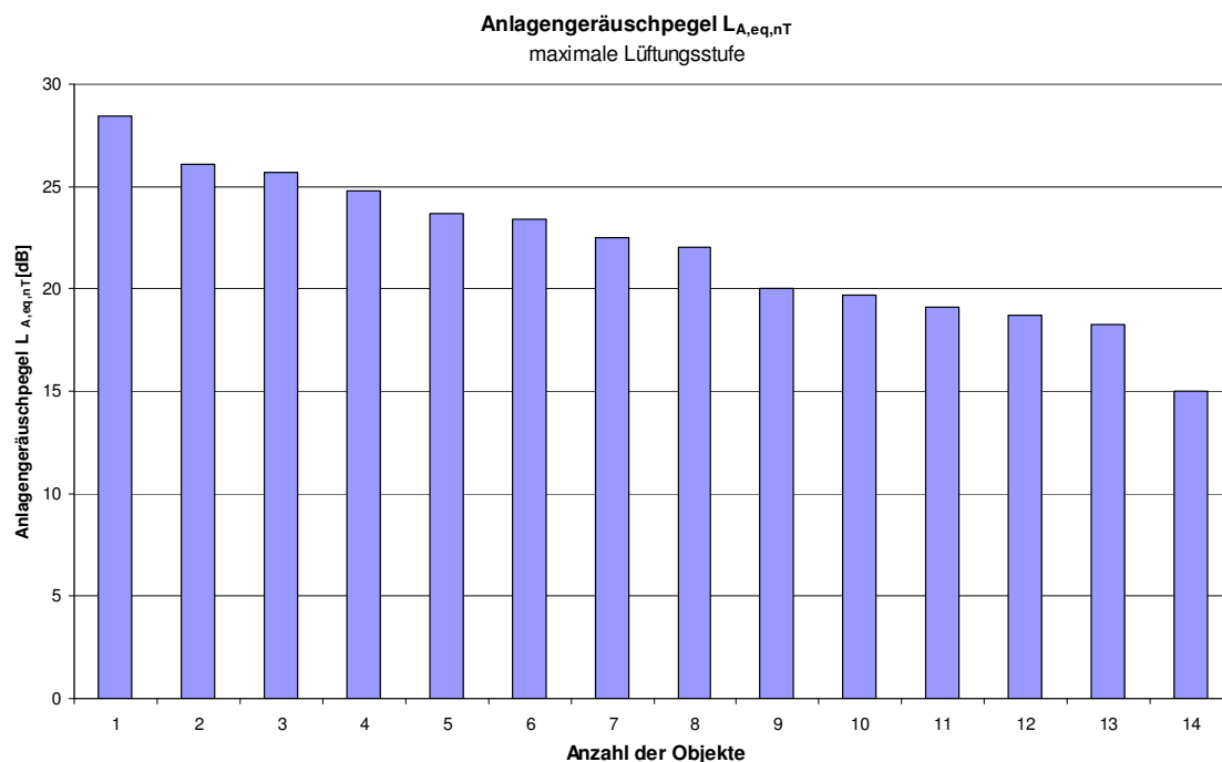
Abb. 3.5.59: Differenz des äquivalenten Anlagengeräuschpegels zwischen ausgeschalteter Anlage und maximaler Lüftungsstufe (Stufe 3) in den Schlafräumen der Objekte mit Wohnraumlüftungsanlage, Ersttermin (M1)
