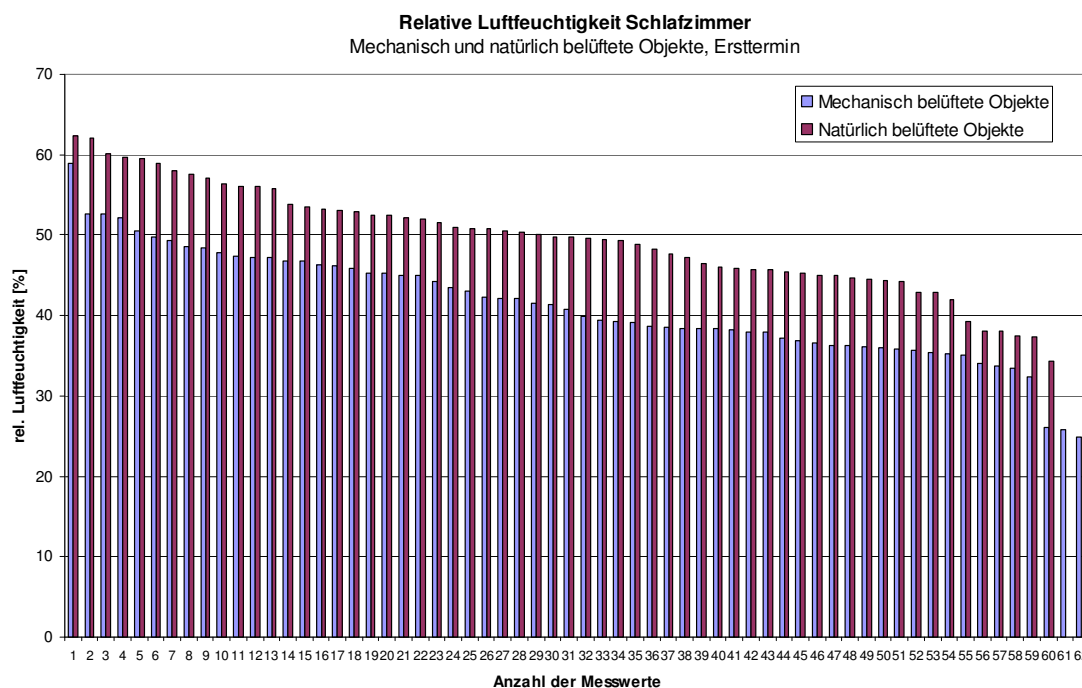
Abb. 3.5.62: Relative Luftfeuchtigkeit im Schlafrum der Objekte mit Wohnraumlüftungsanlage sowie der Objekte mit ausschließlicher Fensterlüftung, arithmetischer Mittelwert über den Zeitraum einer Woche, Ersttermin (M1)
