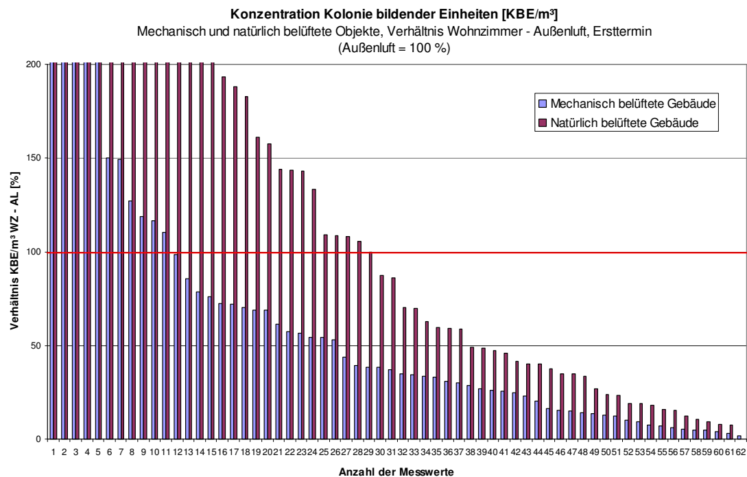
Abb. 3.5.33: Verhältnis der Konzentration an KBE/m 3 in den Wohnräumen der Objekte mit Wohnraumlüftungsanlage sowie der Objekte mit ausschließlicher Fensterlüftung und der Außenluft, Ersttermin (M1)
