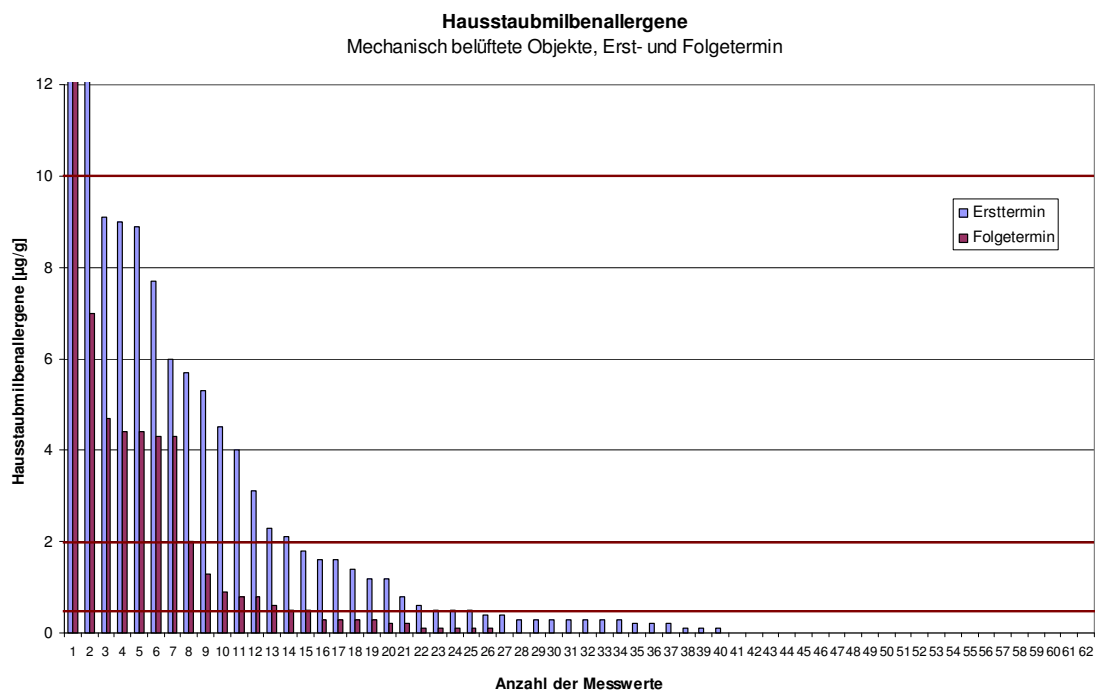
Abb. 3.5.37: Summe der Konzentration an Der p1 und Der p2 in Wohn- und Schlafräumen der Objekte mit Wohnraumlüftungsanlage, Erst- und Folgetermin (M1, M2)
