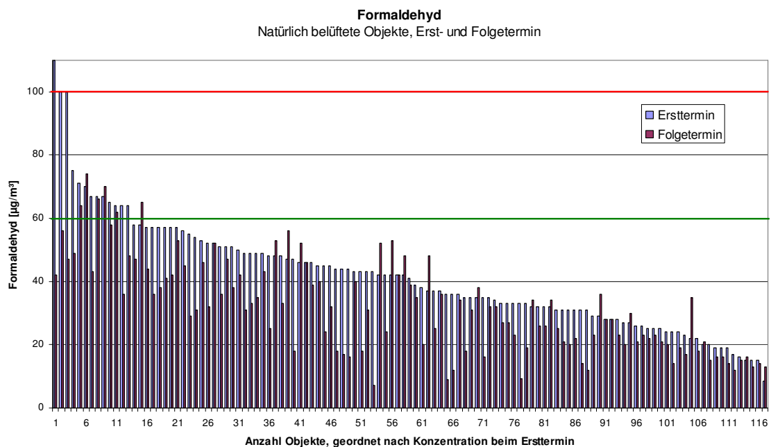
Abb. 4.3.11: Formaldehyd- Konzentrationen in Wohn- und Schlafräumen von Objekten mit ausschließlicher Fensterlüftung, Erst- und jeweils zugeordneter Folgetermin, Veränderung der Konzentrationen, geordnet nach Konzentrationen bei Ersttermin
