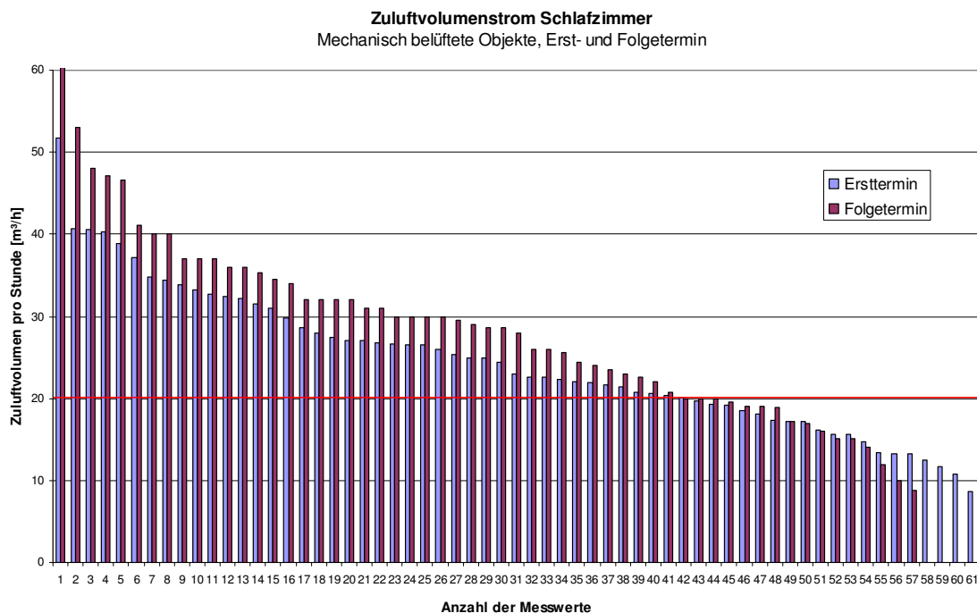
Abb. 3.5.52: Zuluftvolumenstrom gesamt in den Schlafräumen der Objekte mit Wohnraumlüftungsanlage, Erst- und Folgetermin (M1, M2)
