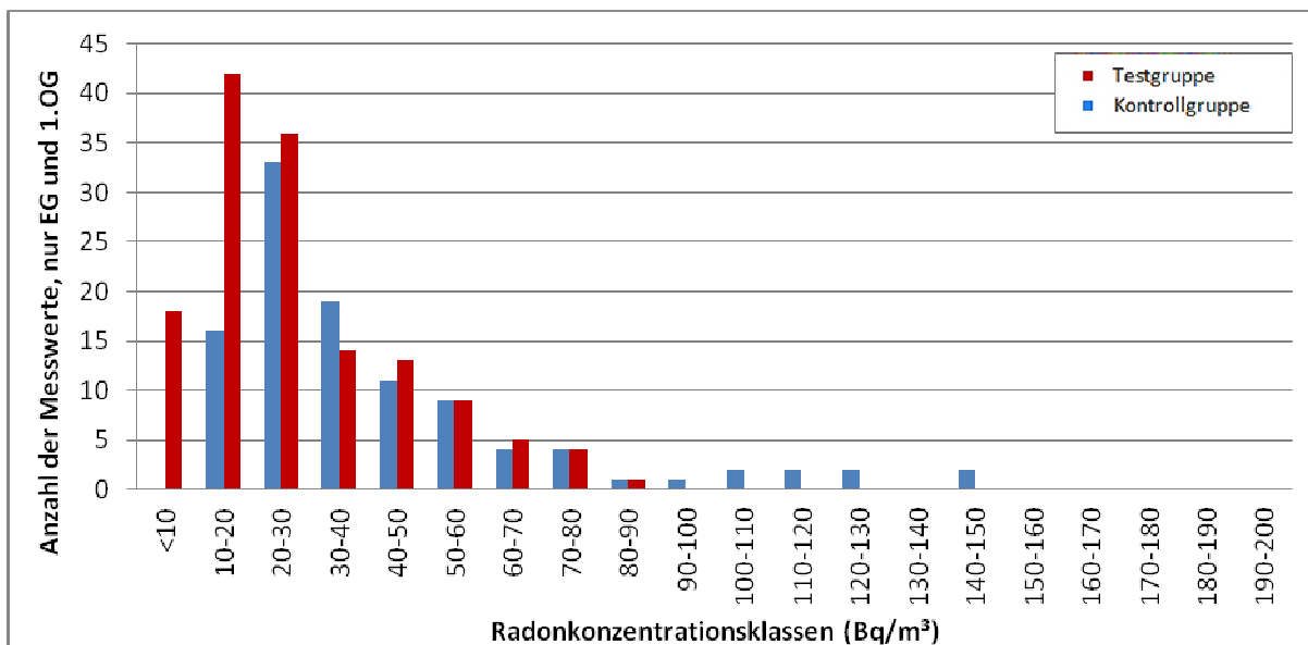
Abb. 8.6: Anzahl der Messwerte in Radonkonzentrationsklassen zu je 10 Bq/m 3 (nur EG und 1.OG von Gebäuden in Gemeinden mit Radonpotenzial \leq 250 Bq/m 3 )
