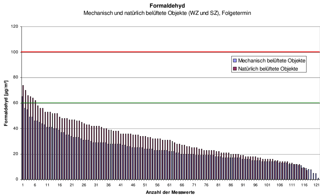
Abb. 3.5.22: Formaldehyd-Konzentrationen in Wohn- und Schlafräumen von Objekten mit Wohnraumlüftungsanlage sowie von Objekten mit ausschließlicher Fensterlüftung, Folgetermin (M2)
