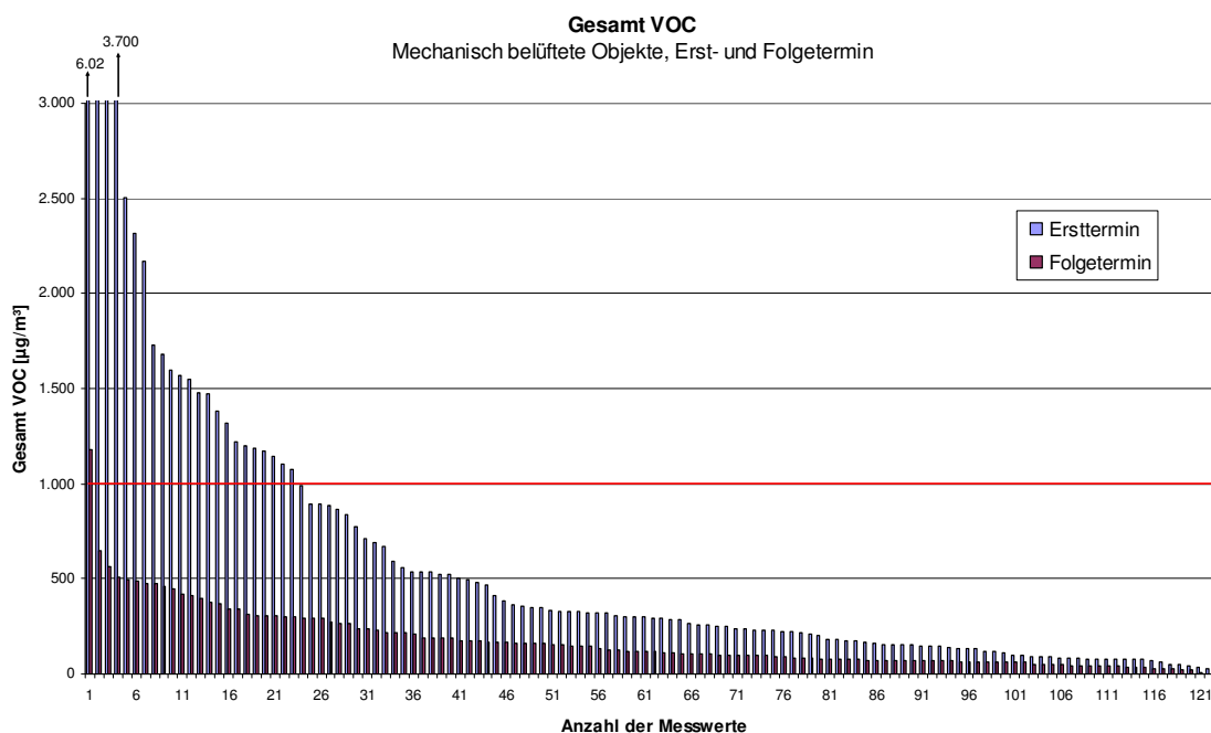
Abb. 3.5.1: Gesamt VOC-Werte in Wohn- und Schlafräumen von Objekten mit Wohnraumlüftungsanlage, Erst- und Folgetermin (M1, M2)
