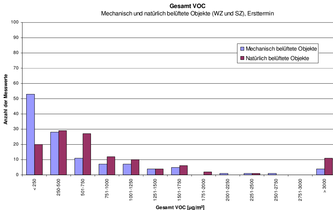
Abb. 4.3.3: Anzahl der Gesamt VOC- Messwerte in Konzentrationsklassen zu je 250 µg/m³, Wohn- und Schlafräume von Objekten mit Wohnraumlüftungsanlage (n=122) und Objekten mit ausschließlicher Fensterlüftung (n=122) Objekte, Ersttermin (M1)
