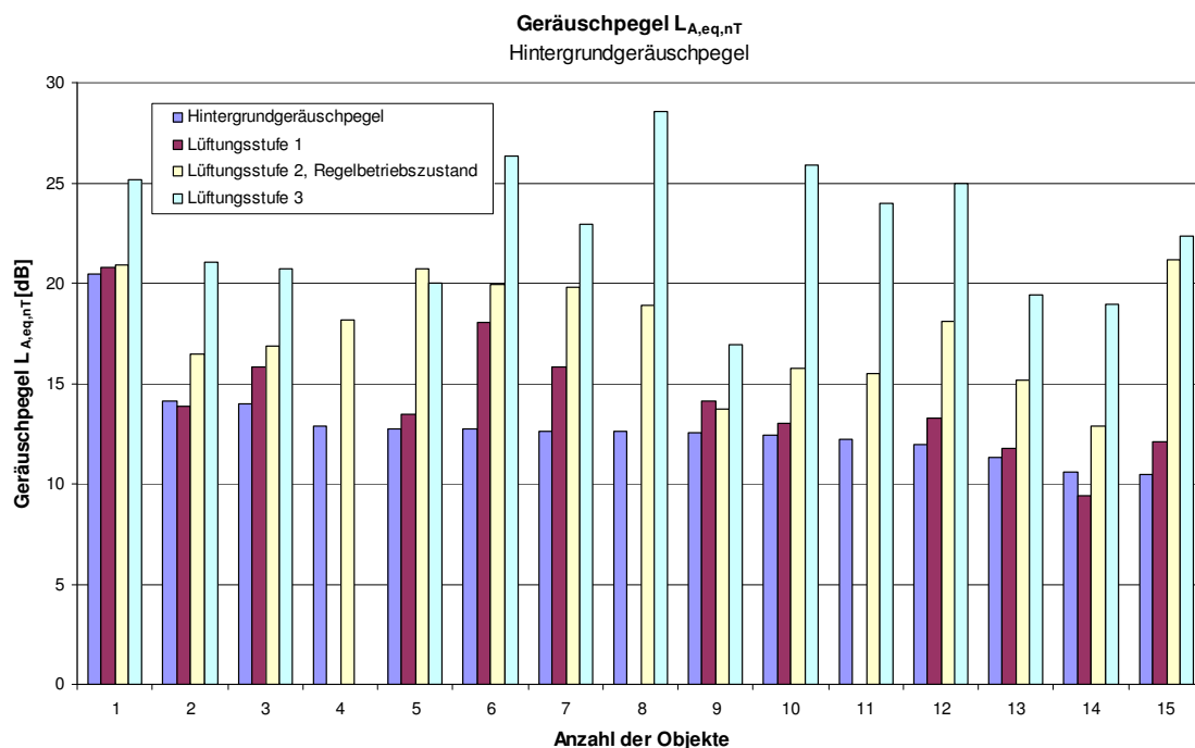
Abb. 3.5.57: Hintergrundgeräuschpegel und äquivalenter Anlagengeräuschpegel in den Schlafräumen der Objekte mit Wohnraumlüftungsanlage, Ersttermin (M1). Es ist ersichtlich, dass für den Regelbetriebszustand (gelber Balken) alle Lüftungsanlagen sowohl die baugesetzlichen Anforderung als auch die Qualitätsstandards von komfortlüftung.at eingehalten werden
