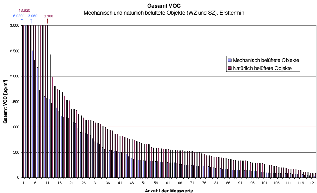
Abb. 3.5.3: Gesamt VOC-Werte in Wohn- und Schlafräumen von Objekten mit Wohnraumlüftungsanlage sowie von Objekten mit ausschließlicher Fensterlüftung, Ersttermin (M1)
