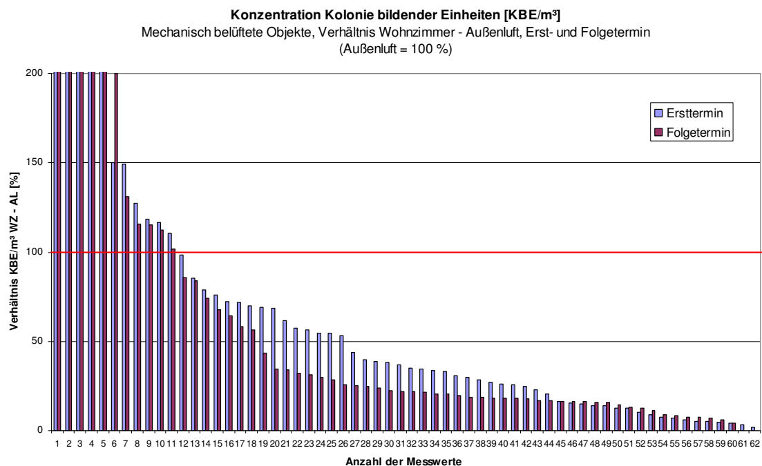
Abb. 3.5.29: Verhältnis der Konzentration an KBE/m 3 in den Wohnräumen der Objekte mit Wohnraumlüftungsanlage und der Außenluft, Erst- und Folgetermin (M1, M2)
