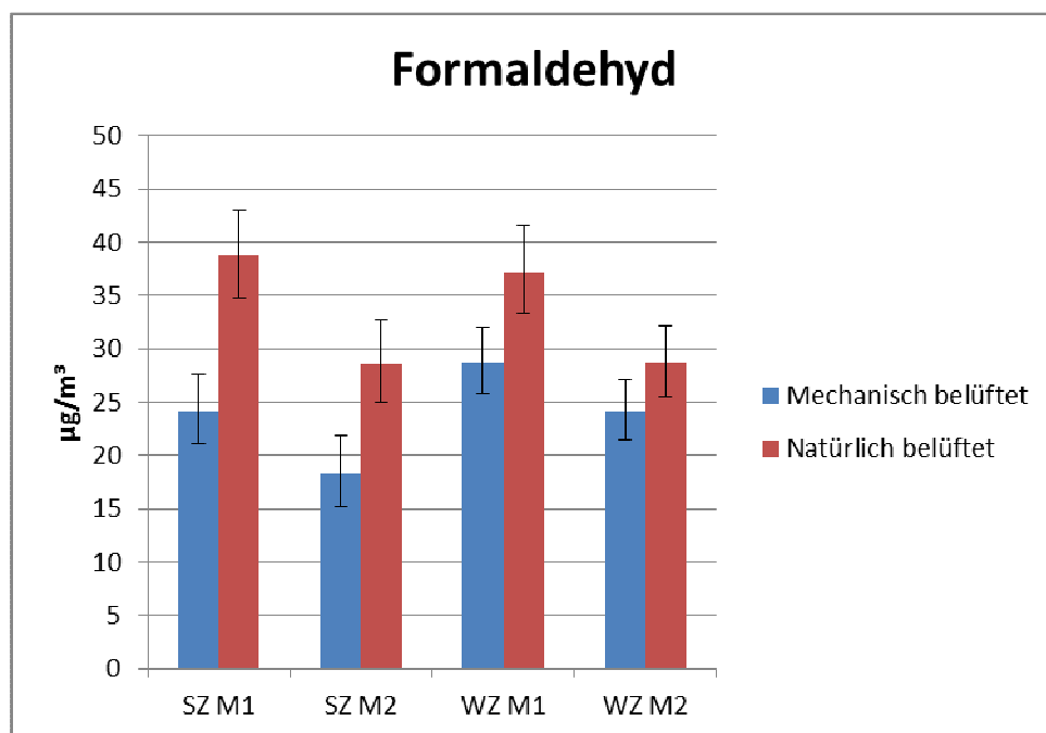
Abb. 4.3.9: Formaldehyd-Werte in Wohn- (WZ) und Schlafräumen (SZ) von Objekten mit Wohnraumlüftungsanlage sowie von Objekten mit ausschließlicher Fensterlüftung, Erst- und Folgetermin (M1, M2), geometrische Mittelwerte und 95 % Konfidenzintervalle
