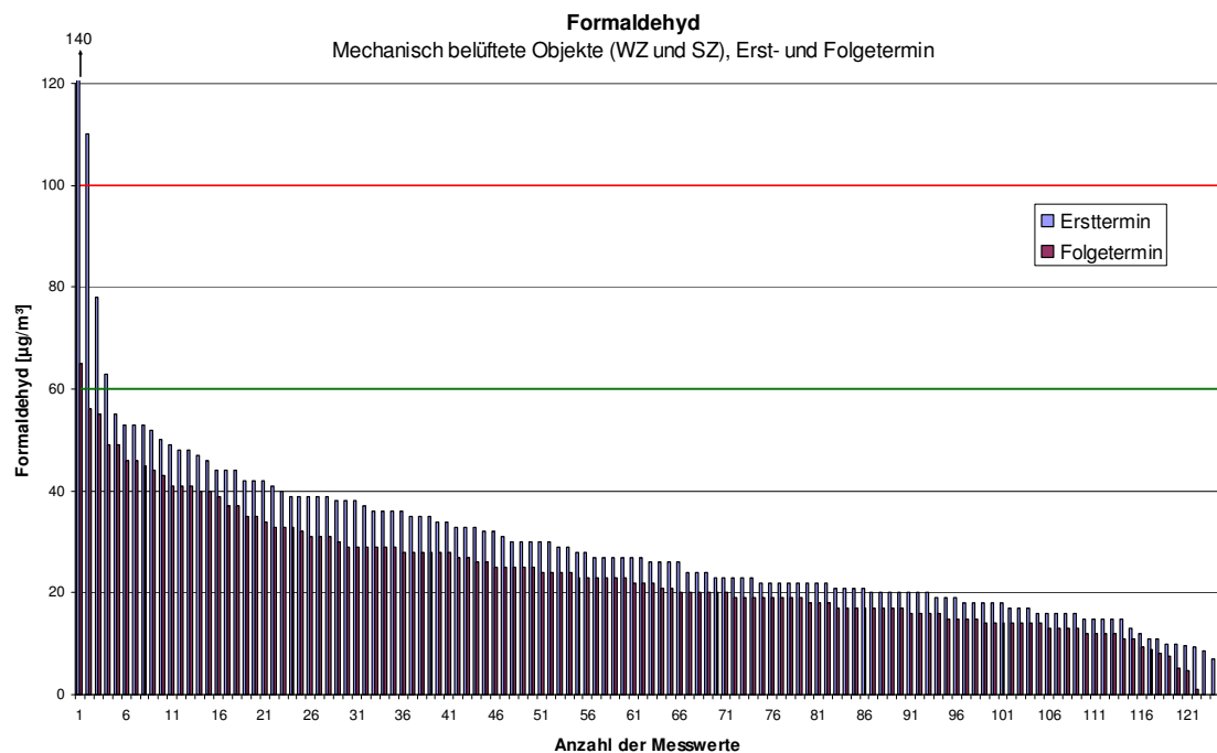
Abb. 3.5.19: Formaldehyd-Konzentrationen in Wohn- und Schlafräumen von Objekten mit Wohnraumlüftungsanlage, Erst- und Folgetermin (M1, M2)
