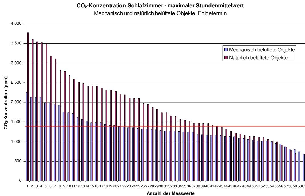
Abb. 3.5.51: CO 2 -Konzentration (max. gleitender Stundenmittelwert) im Schlafraum der Objekte mit Wohnraumlüftungsanlage sowie der Objekte mit ausschließlicher Fensterlüftung, Folgetermin (M2)
