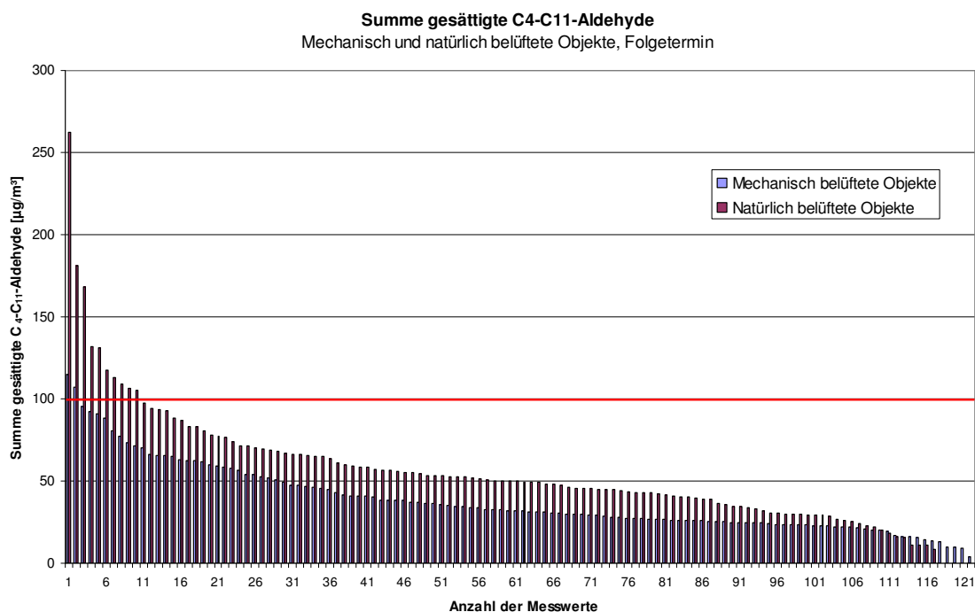
Abb. 3.5.27: Summe gesättigter azyklischer aliphatischer C 4 -C 11 -Aldehyde in Wohn- und Schlafräumen von Objekten mit Wohnraumlüftungsanlage sowie von Objekten mit ausschließlicher Fensterlüftung, Folgetermin (M2)
