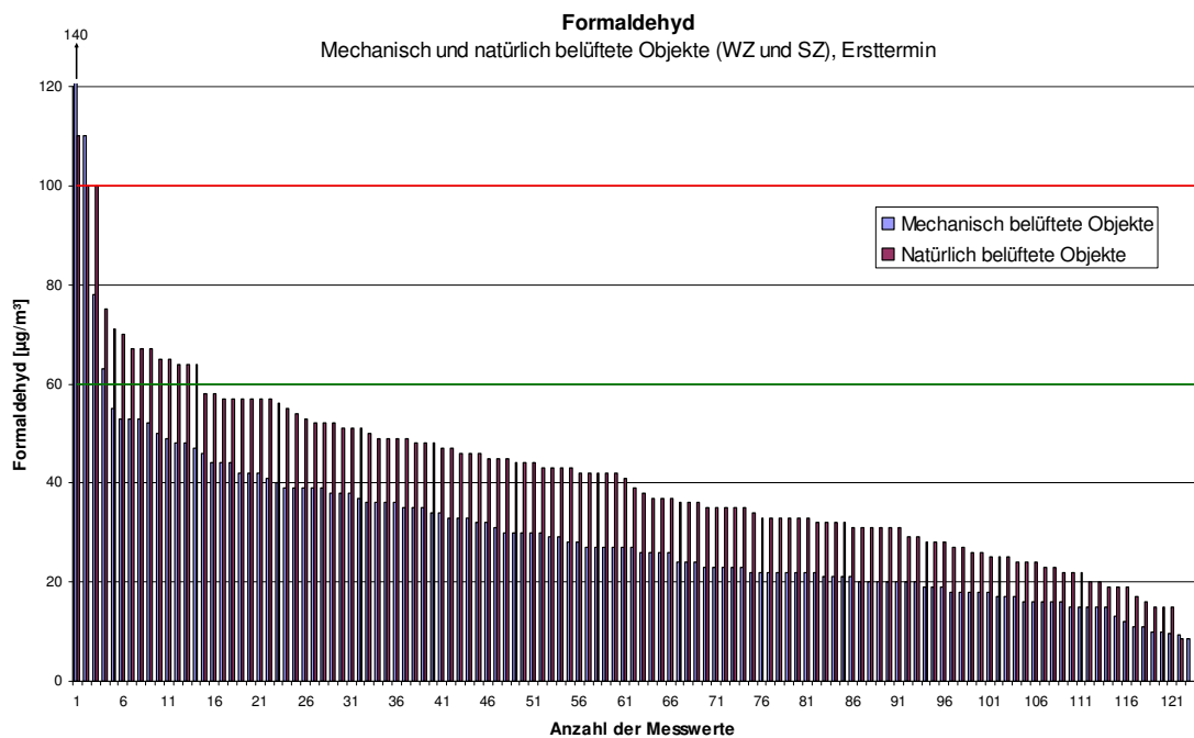
Abb. 3.5.21: Formaldehyd-Konzentrationen in Wohn- und Schlafräumen von Objekten mit Wohnraumlüftungsanlage sowie von Objekten mit ausschließlicher Fensterlüftung, Ersttermin (M1)
