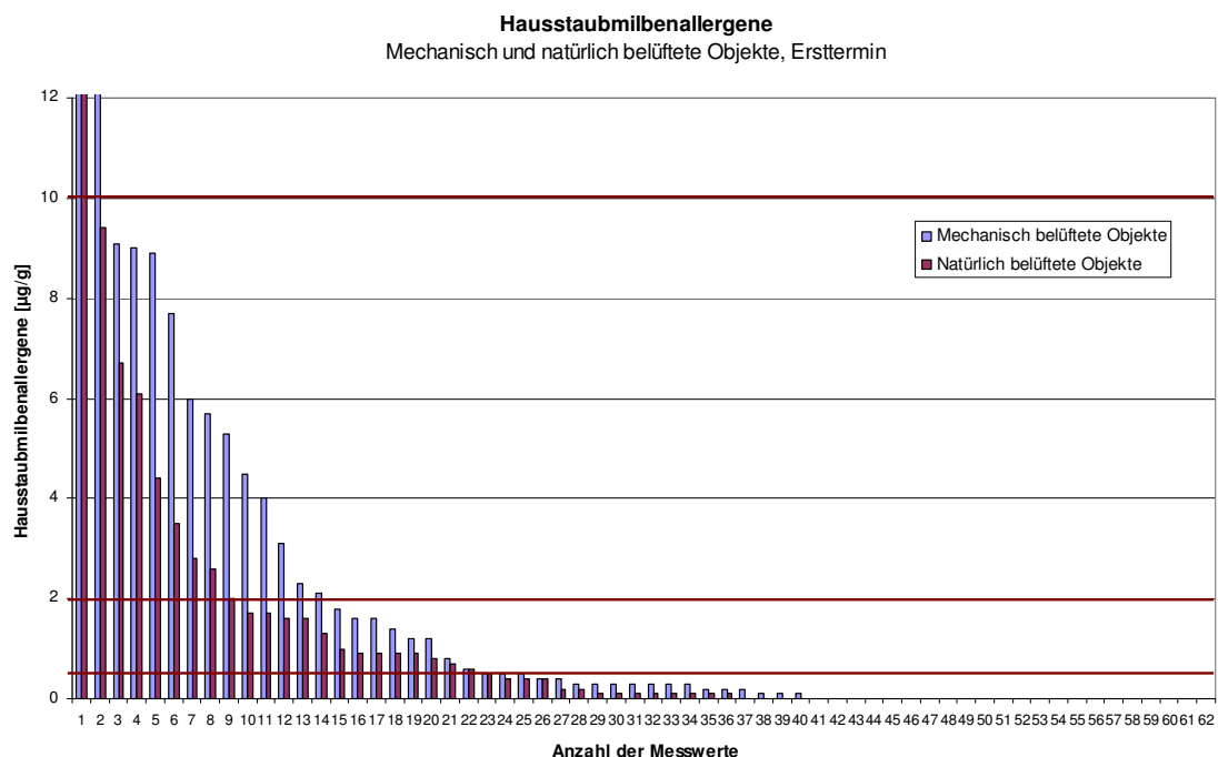
Abb. 3.5.39: Summe der Konzentration an Der p1 und Der p2 in Wohn- und Schlafräumen der Objekte mit Wohnraumlüftungsanlage sowie der Objekte mit ausschließlicher Fensterlüftung, Ersttermin (M1)
