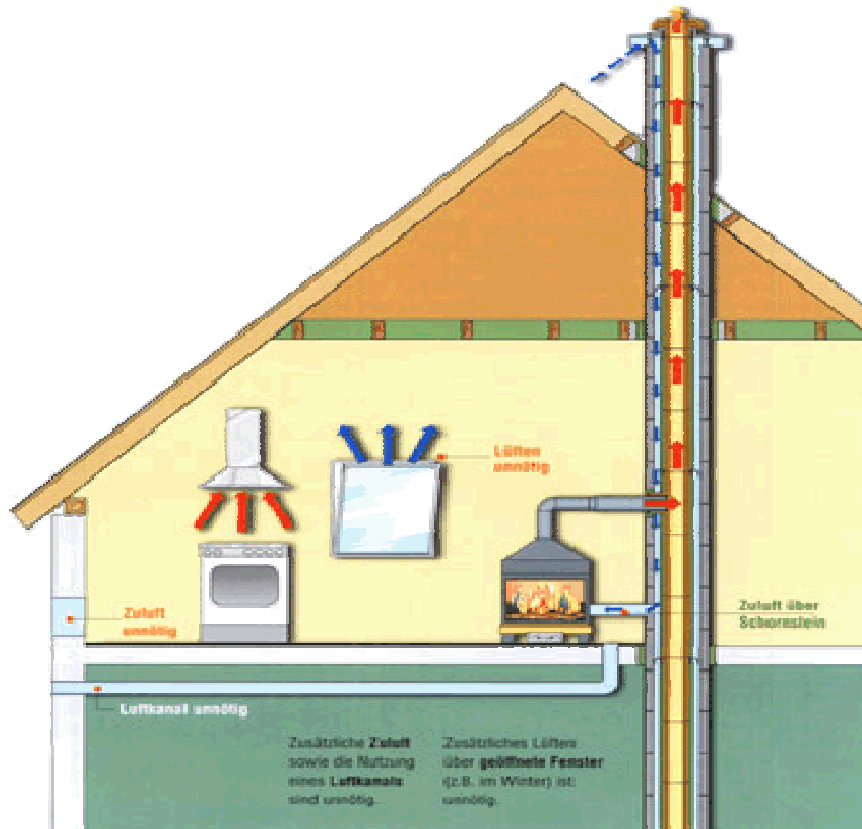
Externe Luftzufuhr über Rohr nach außen oder Kamin
