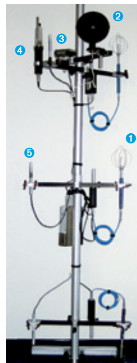
Abbildung 3: Klimamess-System mit verschiedenen Sensoren
