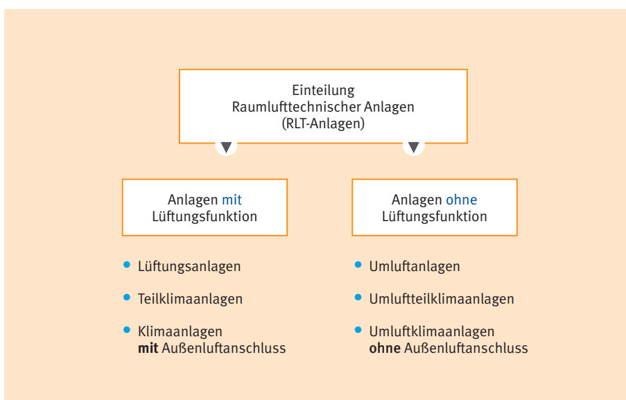
Abbildung 4: Einteilung von RLT-Anlagen
