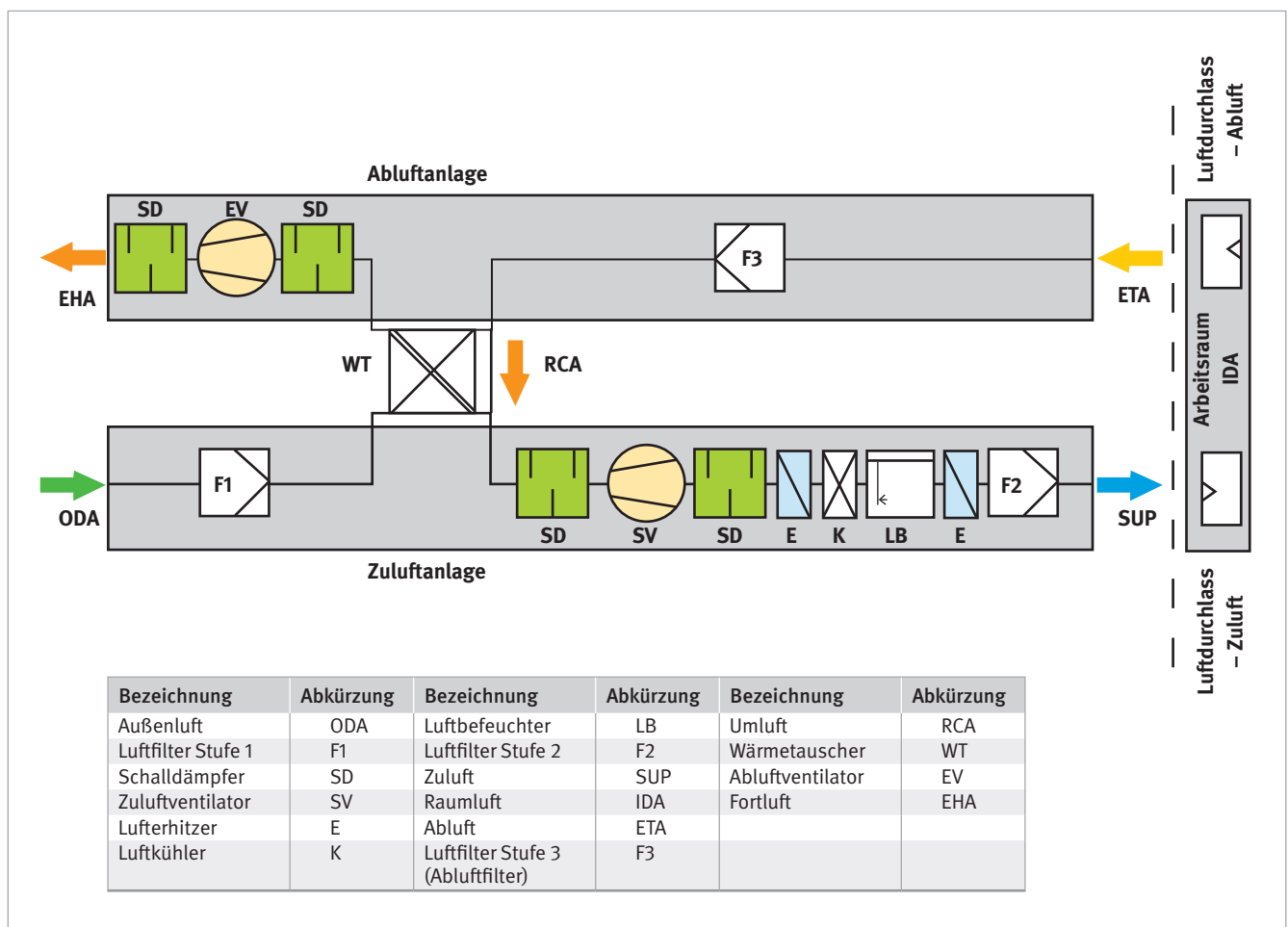
Abbildung 5: Schematischer Aufbau einer RLT-Anlage
